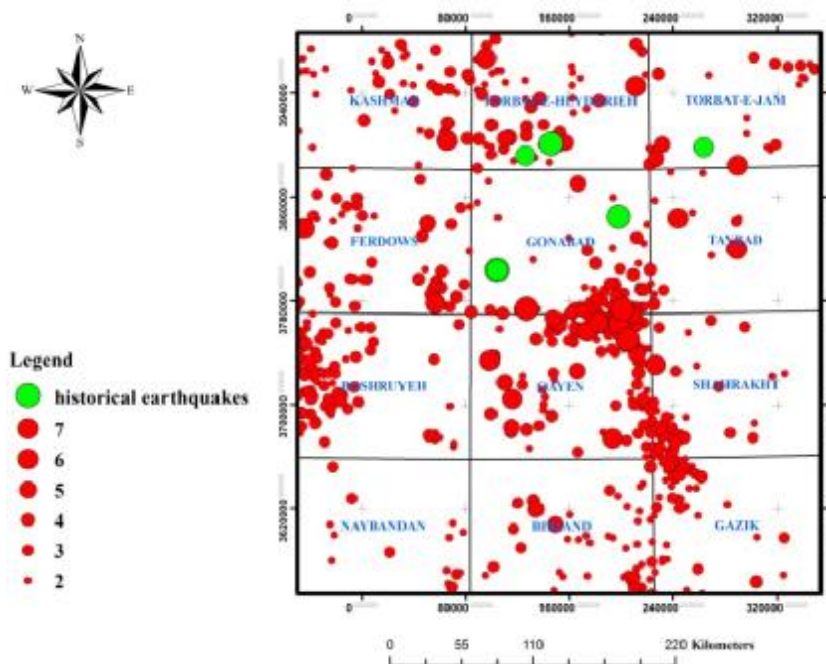
شکل 6: محدوده‌های منطبق بر نقشه‌های زمین‌شناسی 1:250000 به همراه موقعیت زمین لرزه‌ها
