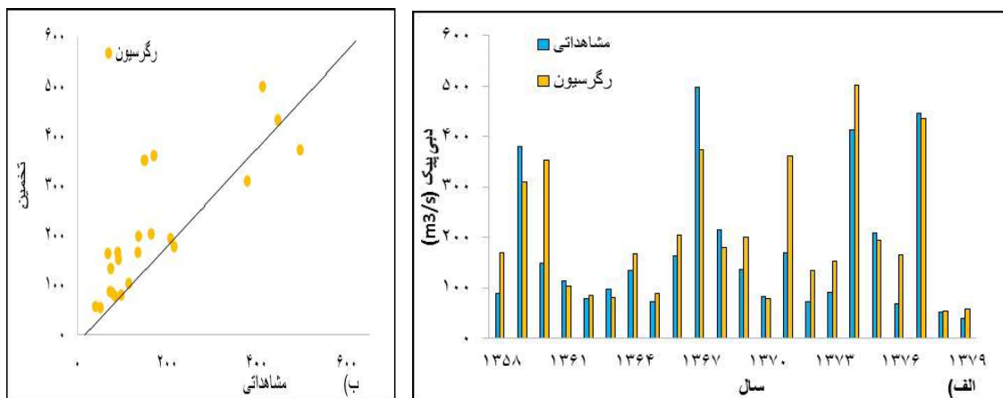
شکل ۳: نمودار الف) مقادیر تخمین زده شده وب) پراکنش مدل مفصل با استفاده از رابطه رگرسیونی
