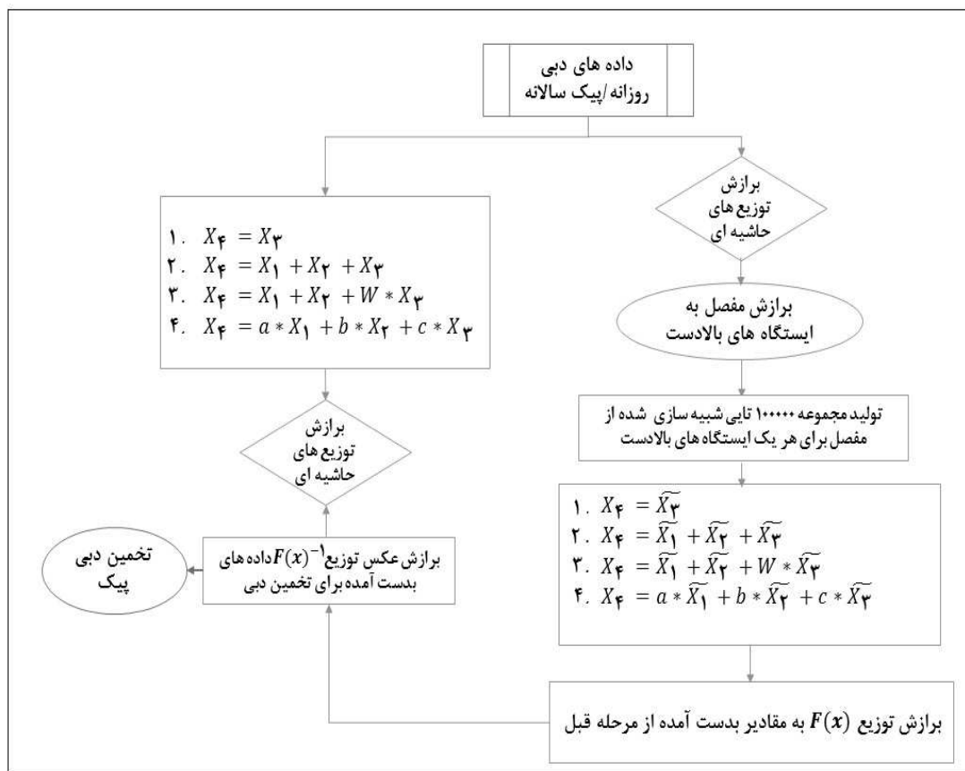
شکل ۲: الگوریتم تحلیل مدل ها، X مقادیر اوج اولیه، \tilde{X} مقادیر دبی شبیه سازی شده
