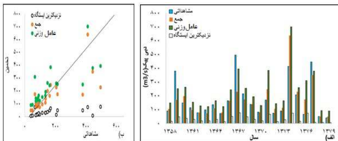
شکل ۴: نمودار الف) مقادیر تخمین زده شده وب) پراکنش مدل مفصل با استفاده از مدل های جمع، عامل وزنی و نزدیکترین ایستگاه
