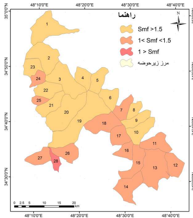
شکل ۱۲: وضعیت شاخص سینوزیترت کوهستان در زیرحوضه‌های توده الوند همدان
