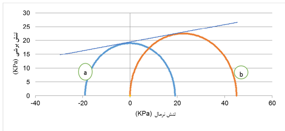
شکل ۶: نمودار رسم شده از نتایج برش پره (a) و پنترومتر (b) مربوط به یک نقطه در اطراف سد سیستان
