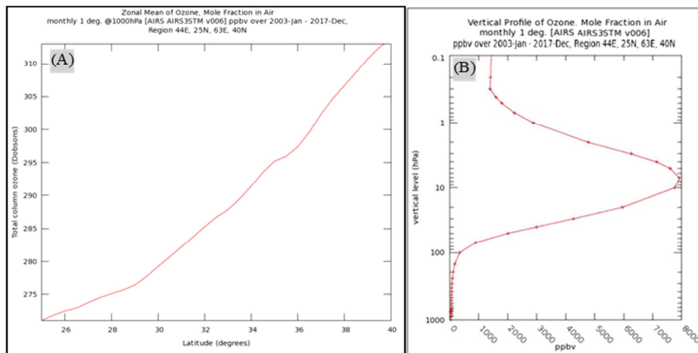
شکل ۱۲: پروفیل قائم توزیع اُزون کلی ستونی در امتداد تراز عمودی ارتفاع ژئوپتانسیل بر فراز ایران (B) – میانگین مداری توزیع اُزون کلی ستونی بر فراز ایران (A) طی دوره آماری (۲۰۰۳ – ۲۰۱۷)
