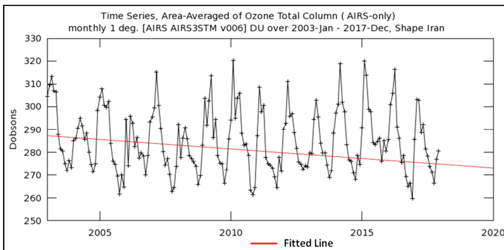
شکل ۳: تغییرات سالانه‌ی آزون کلی ستونی و روند آن بر حسب میانگین ماهانه بر فراز کشور ایران (۲۰۰۳ - ۲۰۱۷)
