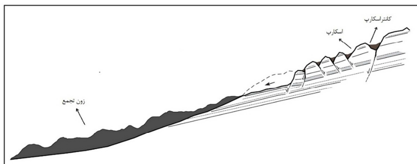
شکل ۱۲: نمایی شماتیک از پدیده رانش زمین (Coquin et al., 2016)
