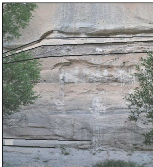
شکل ۱۲: نمایی از پهنه بالائی ایگنیمبریت متنق همراه با پامیس ریزشی که در زیر پهنه ایگنیمبریتی مشاهده می‌شود (دید به سمت جنوب شرقی).
