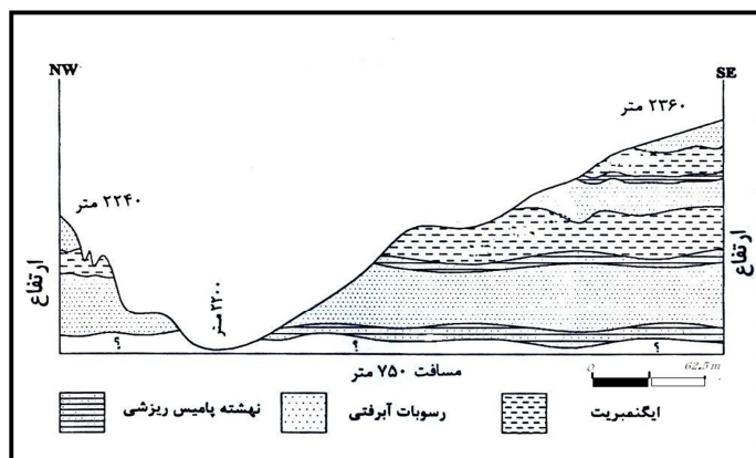
شکل ۱۴: توالی چینه‌شناختی دره متنق در روستای متنق (مقیاس عمودی دقیق نیست).
