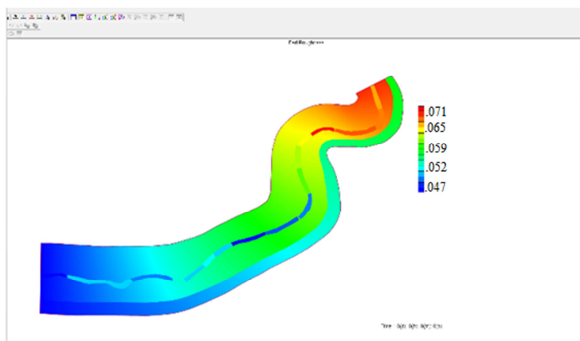
شکل ۳: تنظیم زبری رودخانه در مدل CCHE2D
