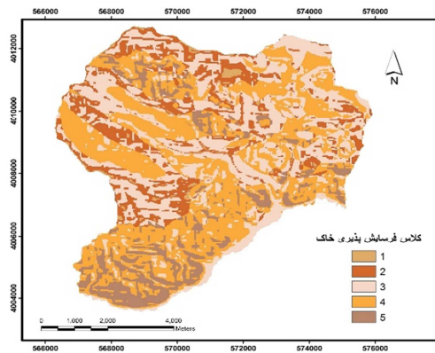
شکل ۱۰: نقشه فرسایش پذیری خاک حوضه بلده
