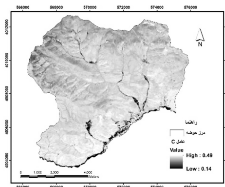
شکل ۶: نقشه فاکتور (C)
