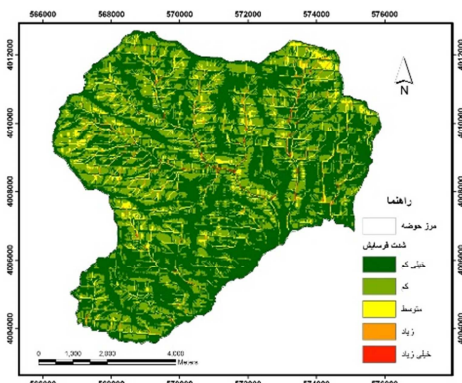
شکل ۷: نقشه شدت فرسایش خاک با مدل RUSLE
