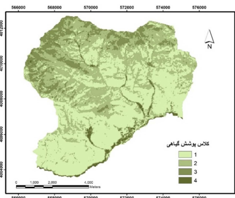
شکل ۱۲: کلاس‌های پوشش گیاهی حوضه بلده
