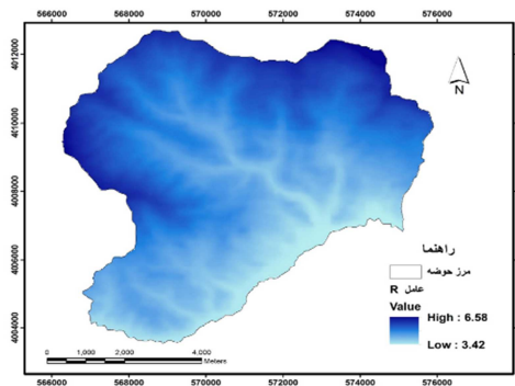
شکل ۳: نقشه فاکتور R
