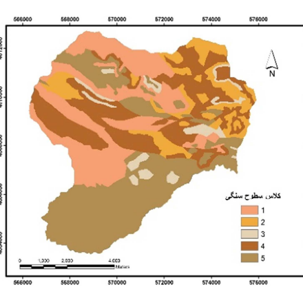
شکل ۹: نقشه کلاس های سنگ شناسی حوضه بلده
