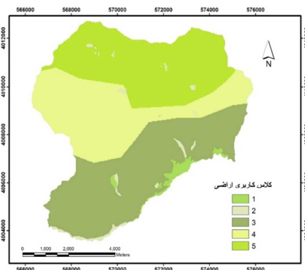
شکل ۱۱: کلاس‌های کاربری اراضی حوضه
