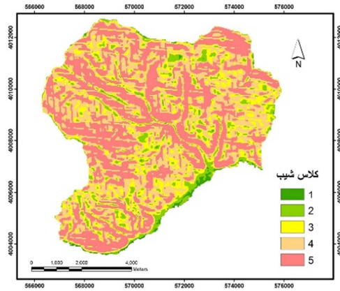
شکل ۸: نقشه کلاس های شیب حوضه بلده
