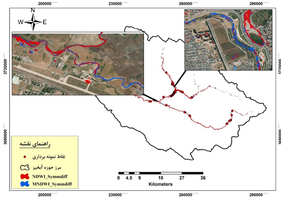
شکل ۴: تعیین پهنه سیل در مسیر جریان با استفاده دو شاخص NDWI و MNDWI
