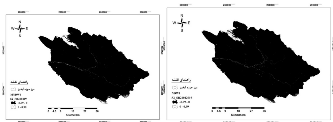
شکل ۳: تفکیک پهنه آبی از سایر اراضی با استفاده از شاخص‌های NDWI و MNDWI تولیدشده از تصاویر سنتینل ۲ پردازش شده در محیط گوگل ارت انجین در تاریخ بعد از سیل ۱۳۹۸ (۲۱-۰۴-۲۰۱۹)
