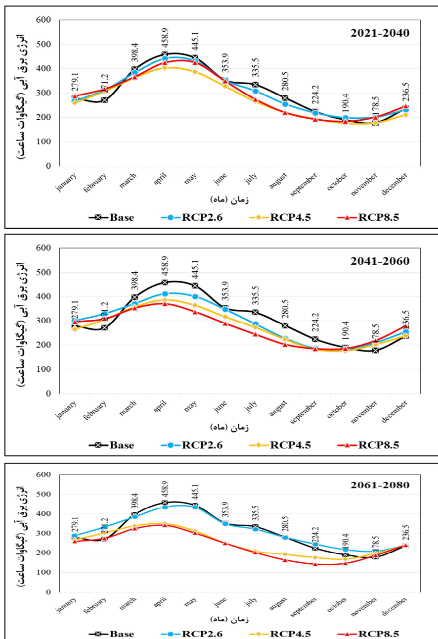
شکل ۵: متوسط بلندمدت ماهانه انرژی برق آبی نیروگاه شهید عباسپور در دوره پایه و دوره‌های آبی و تحت سناریوهای انتشار RCPs
